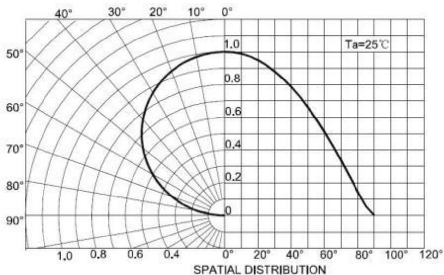
Radiation diagram 辐射图特性曲线
