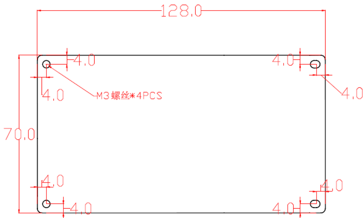
结构尺寸图（单位：毫米）
